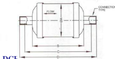
DCH ODS CONNECTION DIMENSIONS
