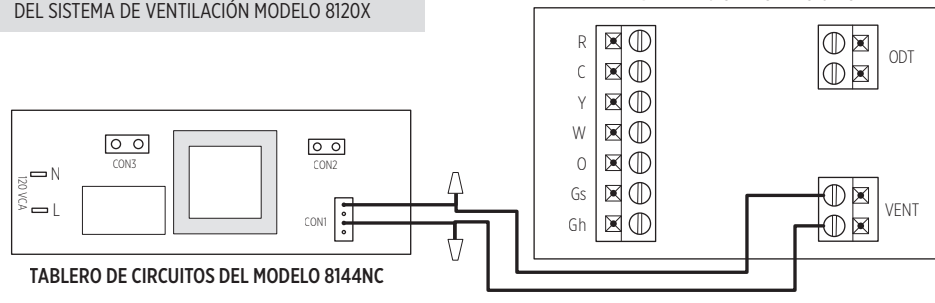
SISTEMA DE CONTROL DIGITAL DEL SISTEMA DE VENTILACIÓN MODELO 8120X
